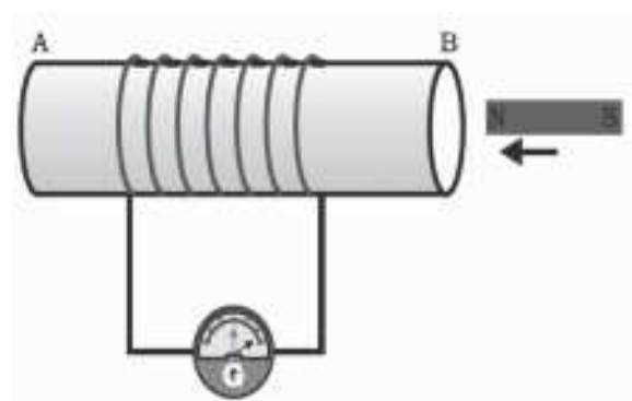
ଚିତ୍ର 9.16 ତୁମ୍ବକଟି କୁଣ୍ଡଳୀ ଆଡ଼କୁ ଗତିକଲେ କୁଣ୍ଡଳୀରେ ବିଦ୍ୟୁତ୍ ସ୍ରୋତ ପ୍ରବାହିତ ହୁଏ। ଏହା ଗାଲ୍ଭାନୋମିଟର ସୂଚୀର ବିକ୍ଷେପ ଦ୍ବାରା ଜାଣି ହେଉଛି।
