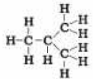
ଚିତ୍ର 4.8 (b) \text{C}_4\text{H}_{10} ସଙ୍କେତ ସହ ଦୁଇଟି ସଂରଚନା ପାଇଁ ସଂପୂର୍ଣ୍ଣ ଅଣୁ
