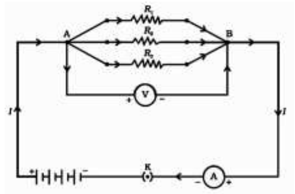
ଚିତ୍ର 8.7 ପ୍ରତିରୋଧର ସମାନ୍ତରାଳ ସଂଯୋଗ
