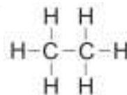
ଚିତ୍ର 4.6 (b) କାର୍ବନ ପରମାଣୁ ସହ ହାଇଡ୍ରୋଜେନ ପରମାଣୁର ବନ୍ଧନ
