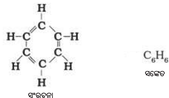
ଚିତ୍ର 4.10 ବେଞ୍ଜିନ୍ର ସଂରଚନା ଓ ସଙ୍କେତ
